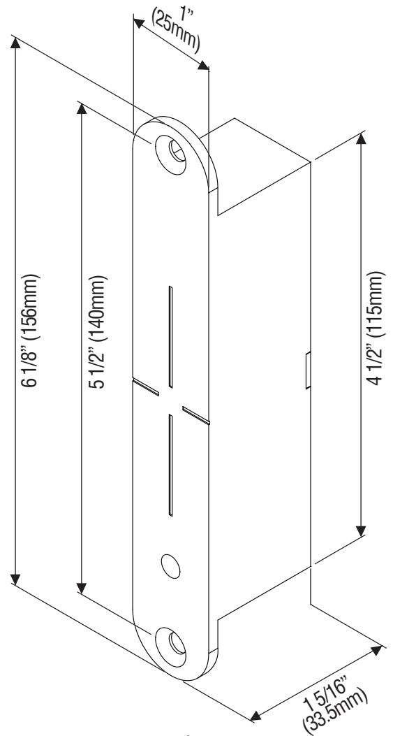
WLP-100 Transmitter
